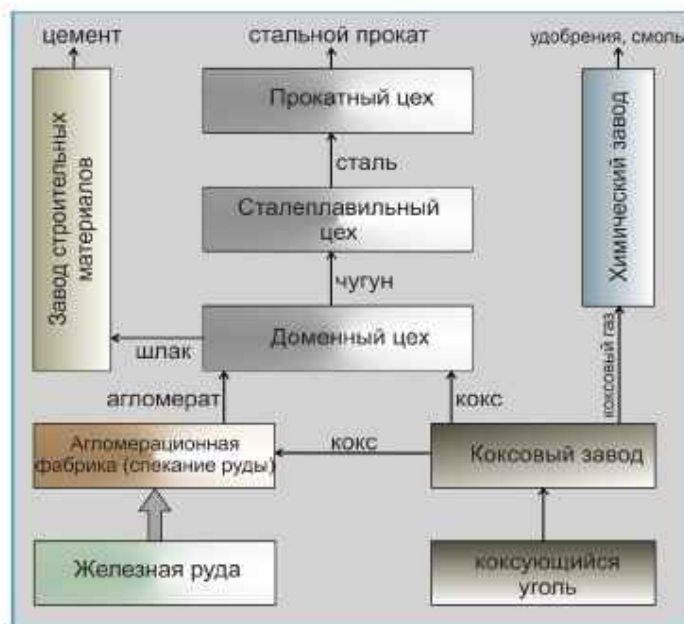
Рис. 208. Схема металлургического комбината
